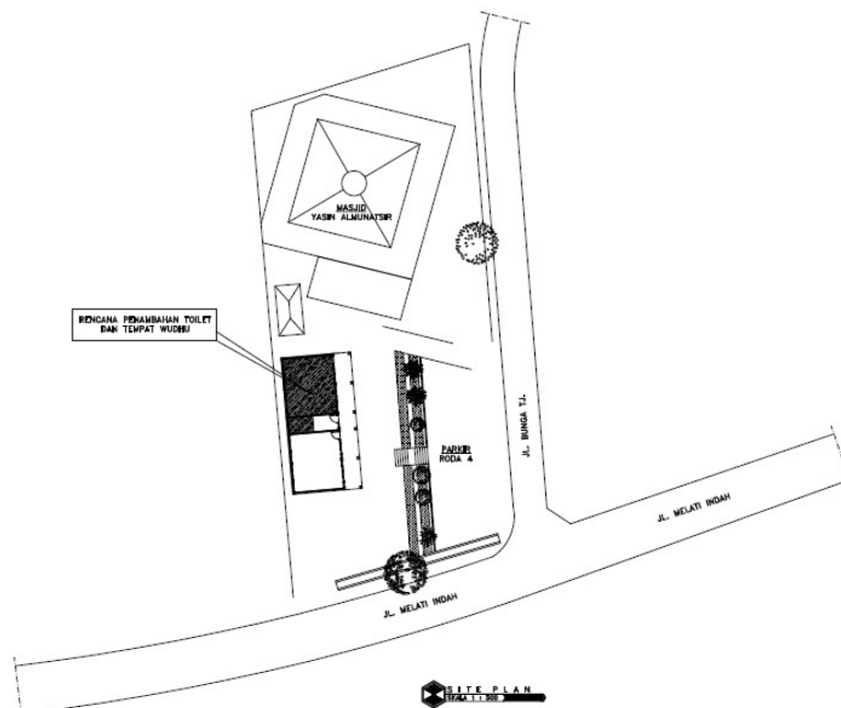
Gambar 5. Site Plan Masjid Yasin Almunatsir
