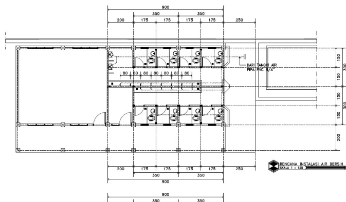
Gambar 12. Denah Instalasi Air Bersih
