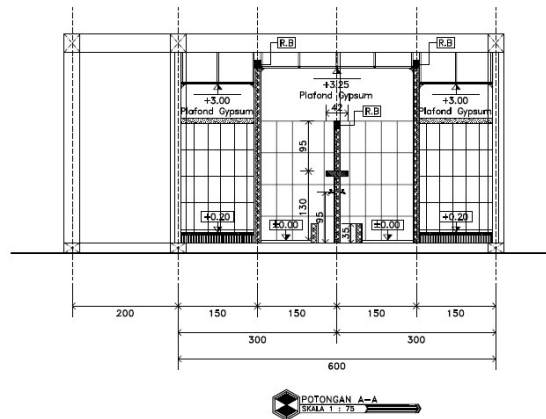
Gambar 9. Gambar Potongan A-A
