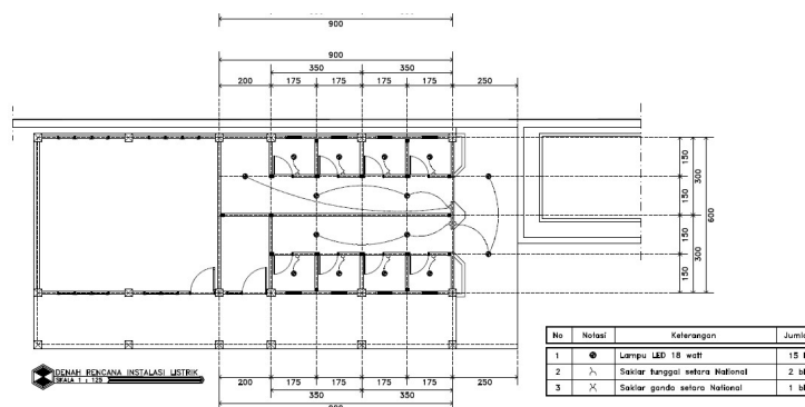
Gambar 11. Denah Rencana Instalasi Listrik
