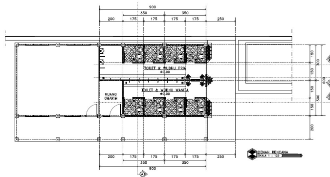
Rencana Gambar 7. Denah
