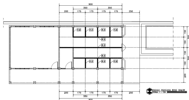
Gambar 10. Denah Rencana Ring Balok
