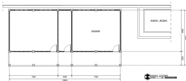
Gambar 6. Denah Eksisting Ruang Kelas pada MDA Masjid Yasin Almunatsir
