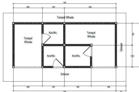
Gambar 2. Denah Eksisting Toilet dan Tempat Wudhu Masjid Yasin Almunatsir
