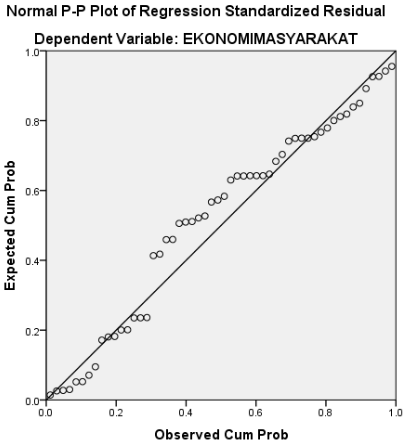
Gambar 4.1 Normalitas Data
