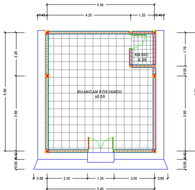
Gambar 4. Denah Rencana Renovasi Posyandu Mekar Kuntum Bau Semerbak
