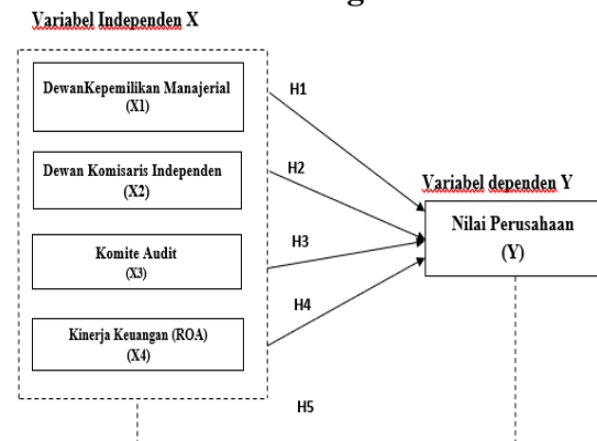
Gambar 2 Kerangka Penelitian
