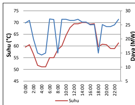
Gambar 5. Grafik Perbandingan Daya Aktif dan Suhu Air
