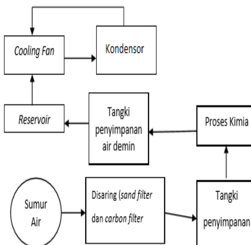
Gambar 1 Sistem kerja cooling fan
