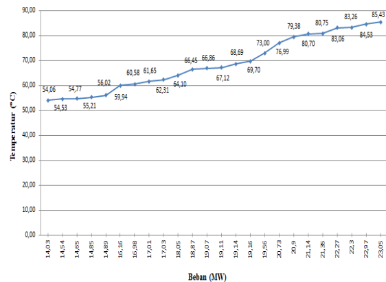
Gambar 6. Grafik Temperatur Terhadap Beban Bulan April.
