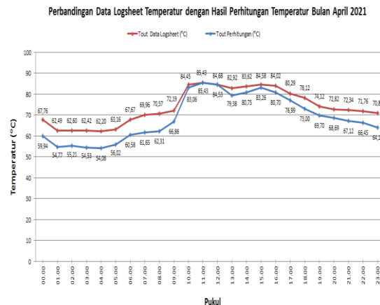
Gambar 8. Grafik Perbandingan Data Logsheets Temperatur dengan Hasil Perhitungan Temperatur Bulan April.
