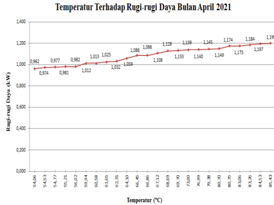
Gambar 5. Grafik Temperatur Terhadap Rugi-rugi Total Bulan April.
