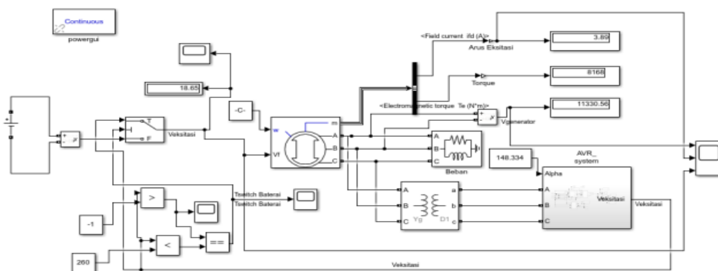
Gambar 10. Simulasi Simulink Generator Sinkron Tiga Phasa pada Pengujian Beban P = 16,16 MW, Q = 1,41 MVAR
