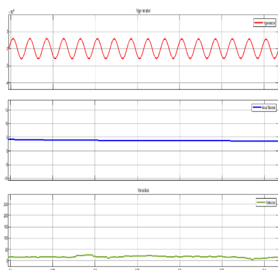
Gambar 11. Gelombang tegangan eksitasi V_f , arus eksitasi I_f , dan tegangan output generator V_{out}
