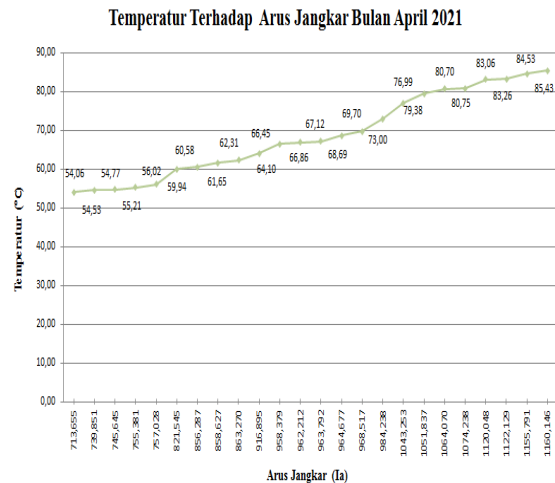
Gambar 7. Grafik Temperatur Terhadap Arus Jangkar Bulan April.
