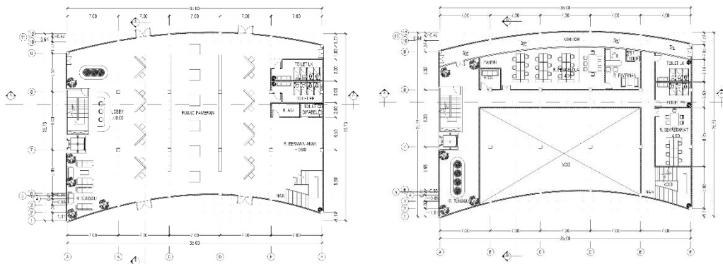
Gambar 14. Denah bangunan utama lt.1 dan 2 (Sumber: data pribadi, 2024)
