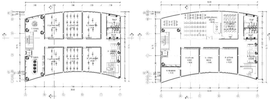
Gambar 15. Denah bangunan utama lt. 3-4 dan 5 (Sumber: data pribadi, 2024)
