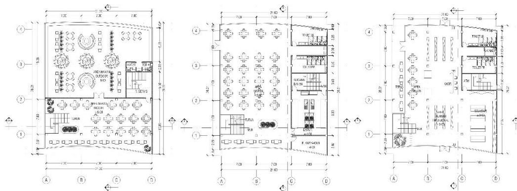
Gambar 16. Denah bangunan komersial lt. 1,2 dan 3 (Sumber: data pribadi, 2024)
