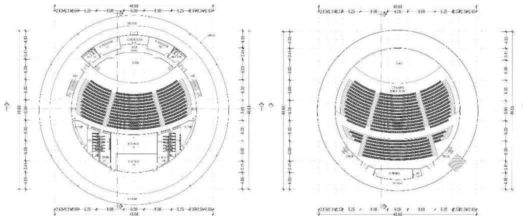
Gambar 4. Denah bangunan teater lt. 1 dan 3 (Sumber: data pribadi, 2024)
