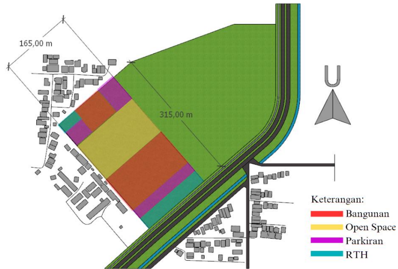
Gambar 2. Zoning tapak (Sumber: data pribadi, 2024)
