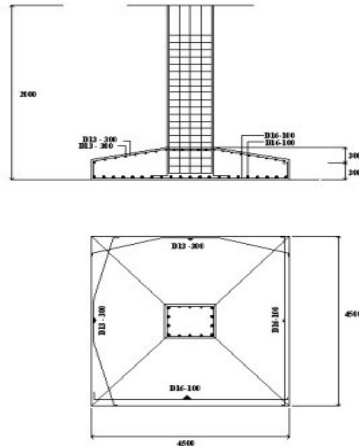
Gambar 14. Pondasi dangkal
