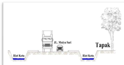
Gambar 4. Potongan Tapak
