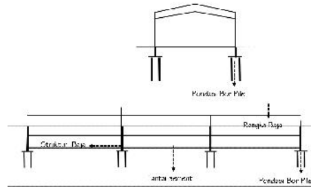
Gambar 13. Struktur bangunan
