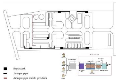
Gambar 14. Sistem Limbah
