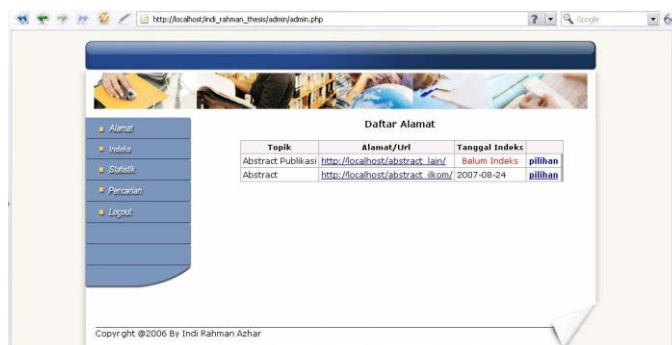
Gambar 4.4 : Antarmuka Alamat
